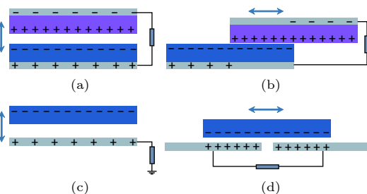
图 3 摩擦纳米发电机的 4 种工作模式 [36] (a) 接触分离式摩擦纳米发电机; (b) 滑动式摩擦纳米发电机; (c) 单电极模式摩擦纳米发电机; (d) 独立层式摩擦纳米发电机
